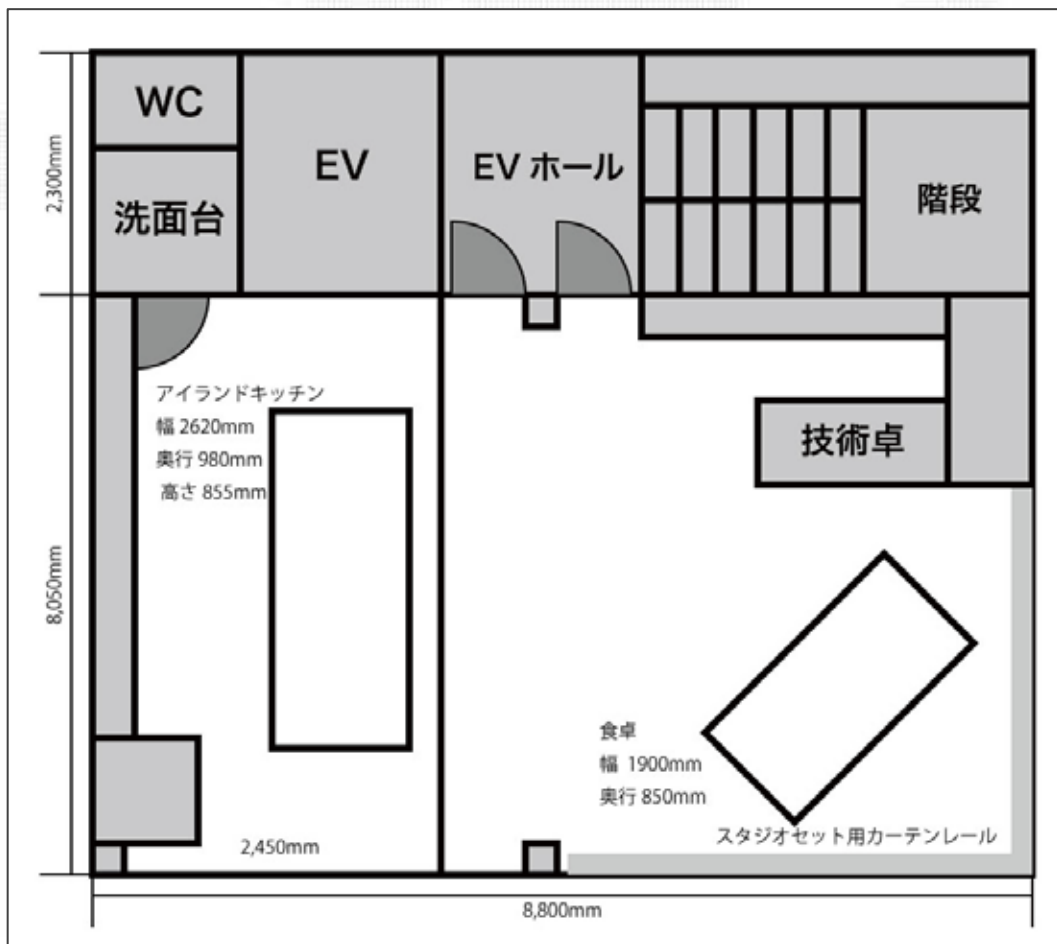
5F キッチンフロア 間取り・レイアウト例
